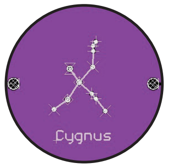
白鳥座
