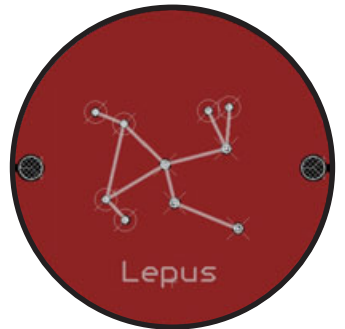
うさぎ座
